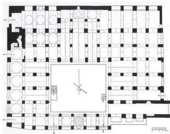
تصویر ۳. پلان مسجد جامع نایین (پیرنیا، ۱۳۸۹: ۱۴۷)
