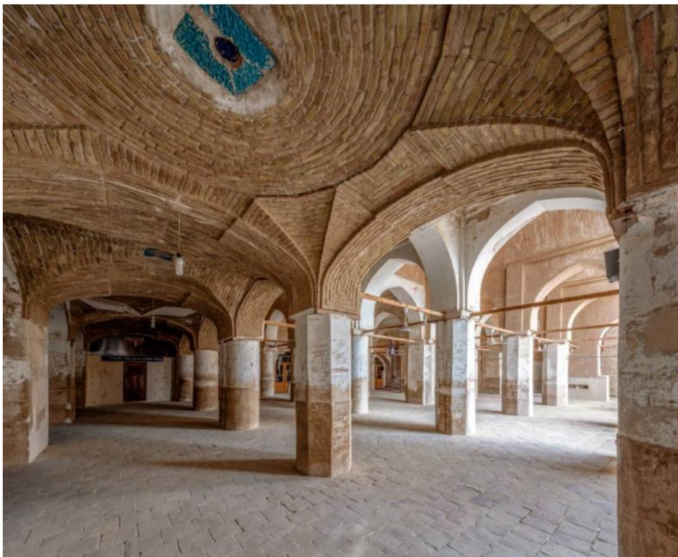
تصویر ۱۳. نمای شبستان مسجد جامع نایین
