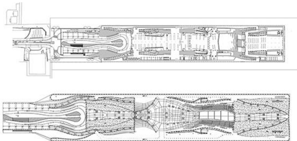
تصویر ۲: پلان طبقه اول و عرشه پایانه دریایی یوکوهاما، (Allen et al, ۲۰۱۷)
