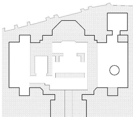
تصویر شماره ۶: پلان سردابه گنبد سلطانیه
