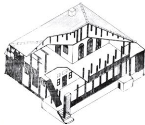
تصویر ۱: غلار گرد در خانه روستایی کپلان (هنج: فرج الهی راد، ۱۳۸۷: ۱۱۷).
