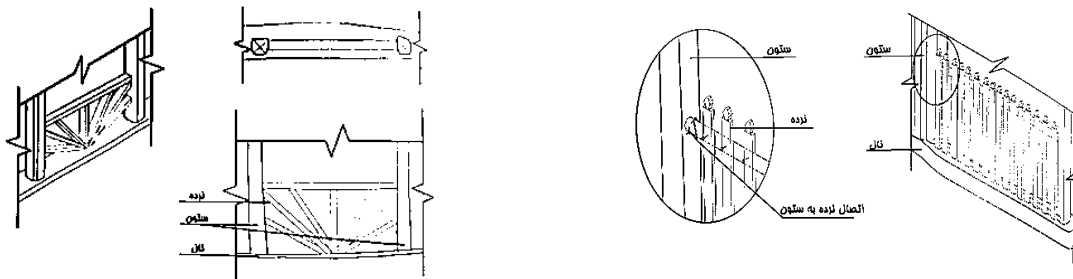
تصویر ۹: جزئیات اجرای نرده کرسی (منبع: طالقانی، ۱۳۸۹: ۸۵). تصویر ۱۰: جزئیات اجرای نرده در تار (منبع: طالقانی، ۱۳۸۹: ۸۵).
