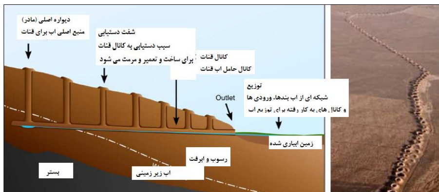
شکل ۶. (سمت چپ) شیوه حفر چاه ها و (سمت راست) طراحی ردیفی چاه
