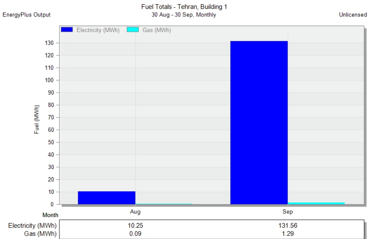
تصویر ۱: نمودار برق مصرفی مرکز خرید یاس از ۳۰ آگوست تا ۳۰ سپتامبر ۲۰۱۹، شبیه‌سازی با نرم‌افزار دیزاین بیلدر (منبع: نگارنده)
