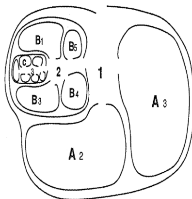
تصویر ۶: ساختار خطه در شهرهای اولیه اسلامی (منبع: Akbar, Jamel, 1990: 22-32)
