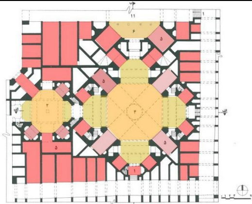
تصویر ۱۴-الف-پلان تیمچه شیخ کاظم، ماخذ: حاجی قاسمی، ۱۳۸۳: الف: ۱۲۰
