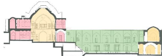
تصویر ۱۱ب-برش تیمچه و سراسر بخشی، ماخذ: (حاجی قاسمی، ۱۳۸۳:ب:۸۳)
