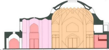
تصویر ۱۷ ب-برش قیصریه، ماخذ: حاجی قاسمی، ۱۳۸۳ الف: ۱۷۳
