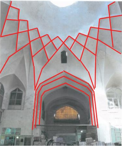
تصویر ۱۷-ج-سقف قیصریه، ماخذ: حاجی قاسمی، ۱۳۸۳ الف: ۱۷۴
