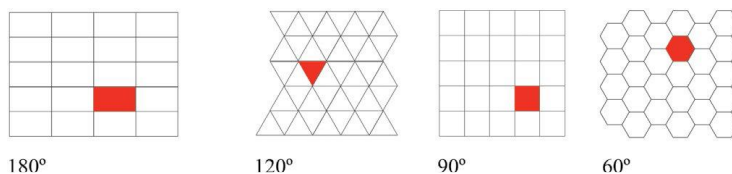
تصویر ۸- نمونه خود متشابهی و تکرار شوندگی هندسی فرکتالی، منبع: زاپولا، ۲۰۰۸
